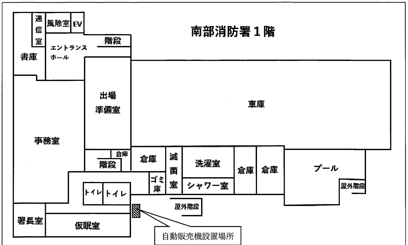
施設平面図
