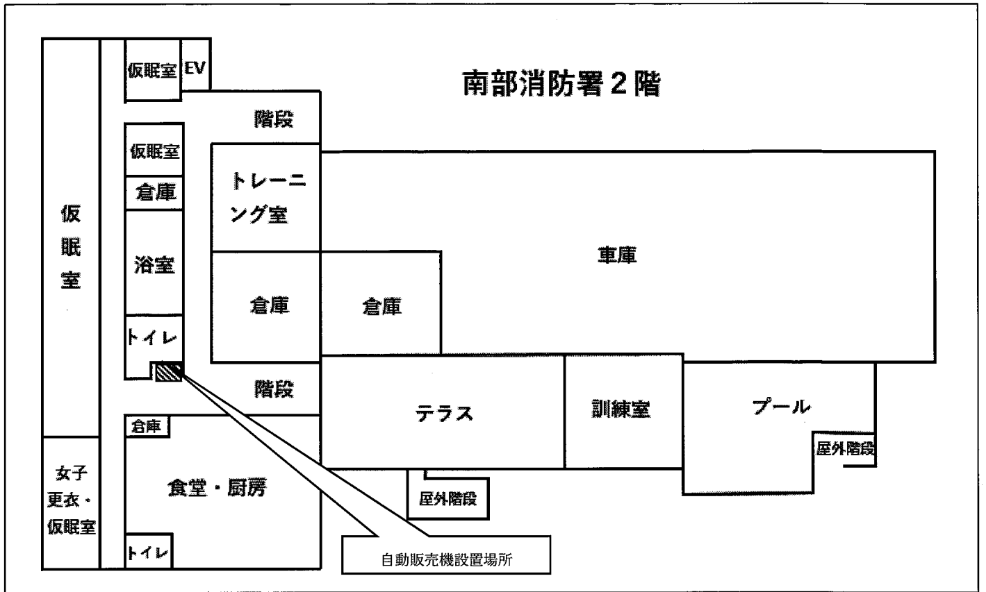
施設平面図
