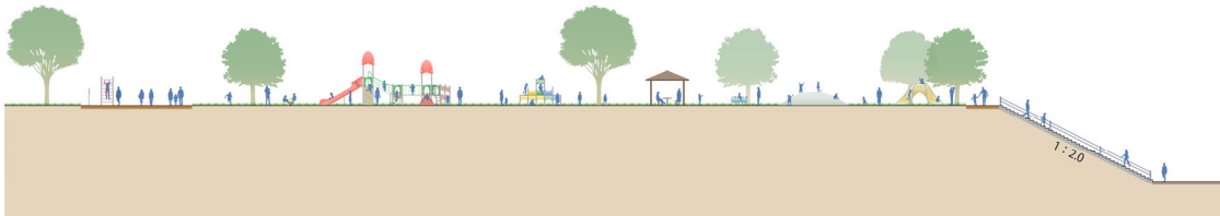
断面①
