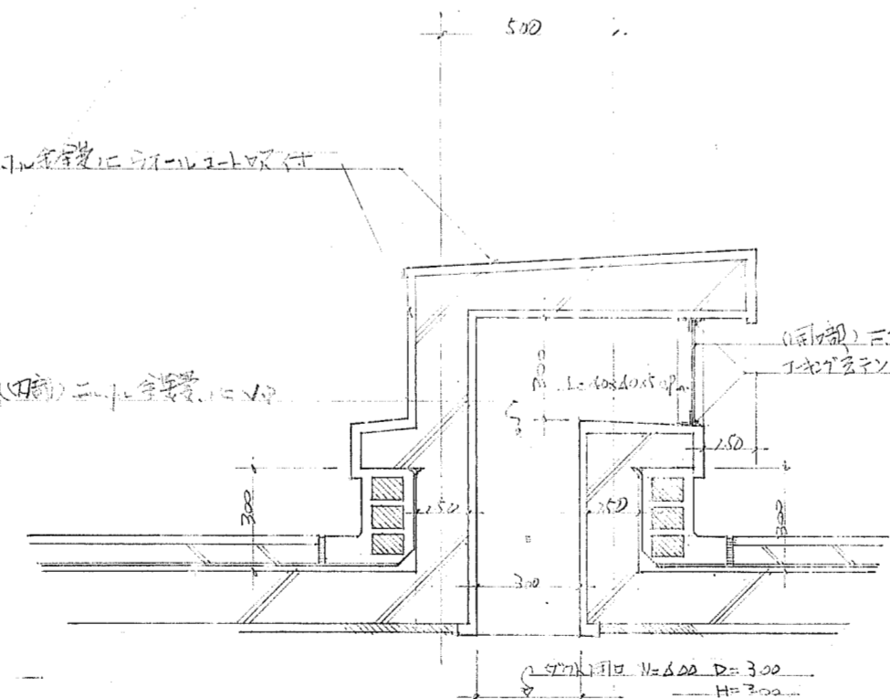
A-A 詳細図 S:1/20
