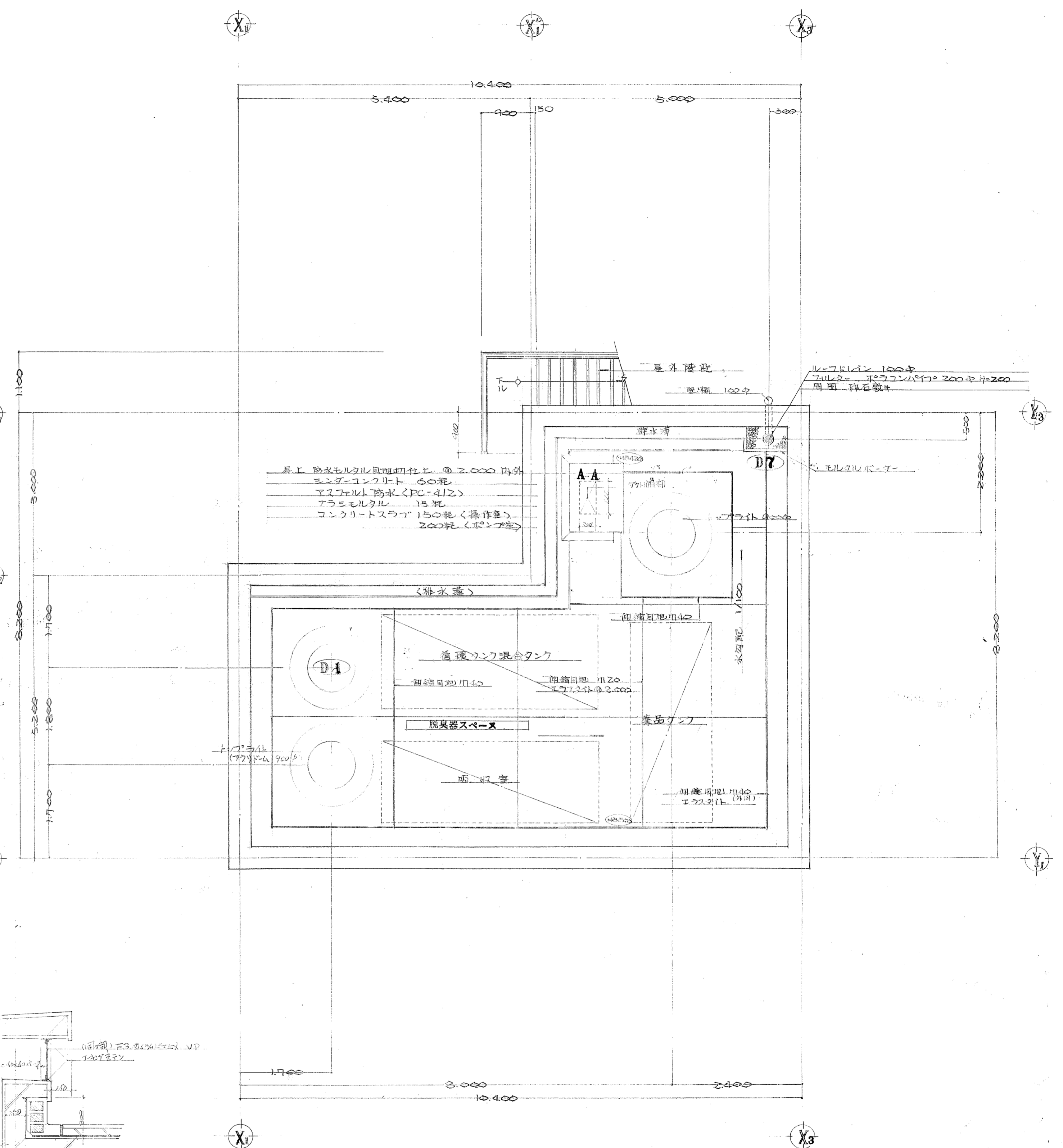
平面図 1:50 +45.420 ~ +45.500
