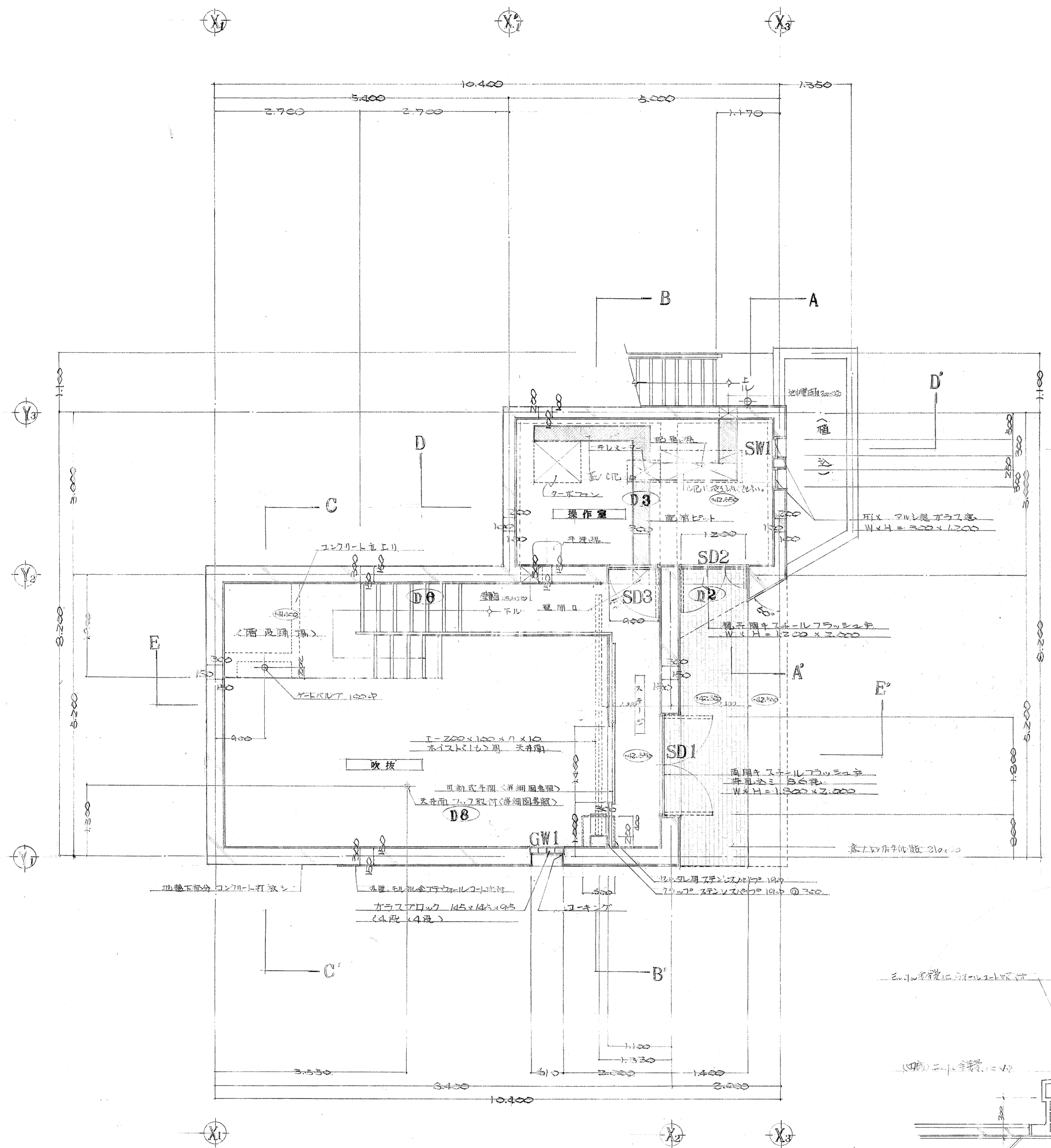
平面図 1:50 +41.400 ~ +42.650
