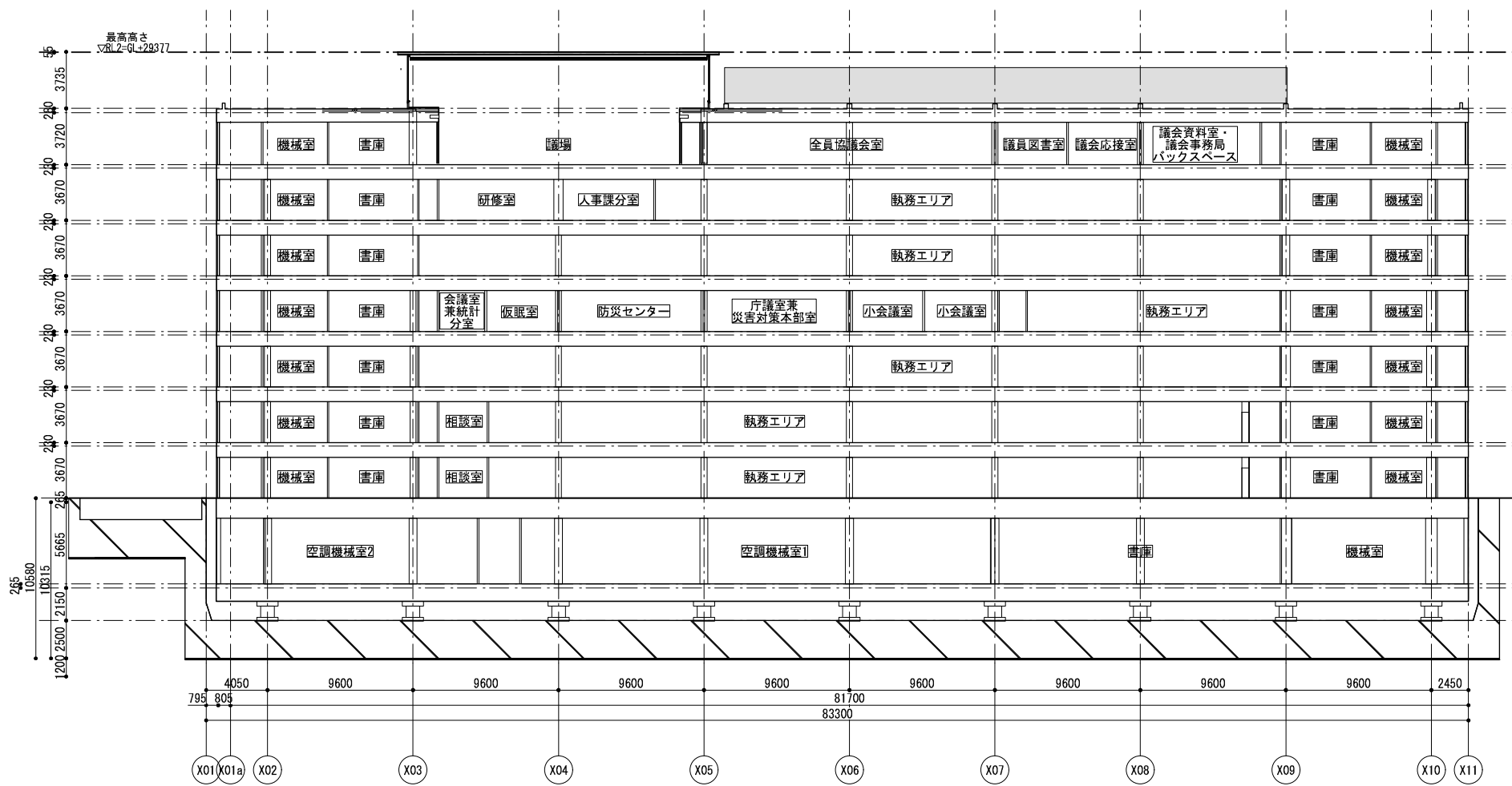
B-B' 断面図
