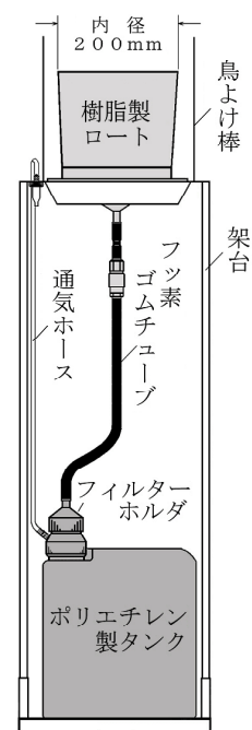
酸性雨ろ過式採取装置
