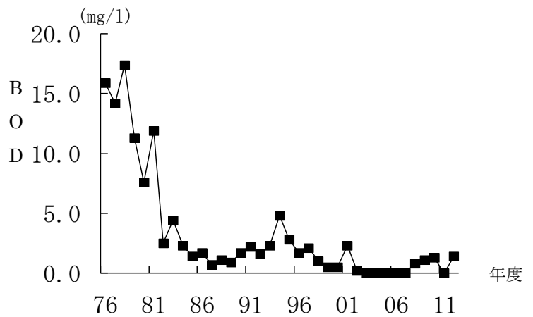
図1-8 BODの経年変化(桜川)
