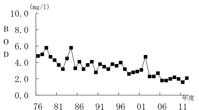
図1-10 BODの経年変化(茂宮川)
