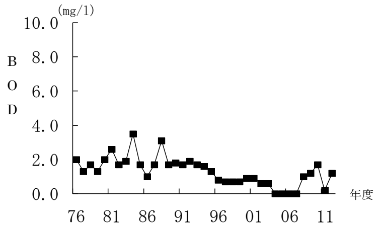
図1-6 BODの経年変化 (東連津川)
