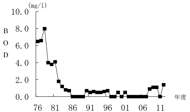
図1-7 BODの経年変化 (鮎川)
