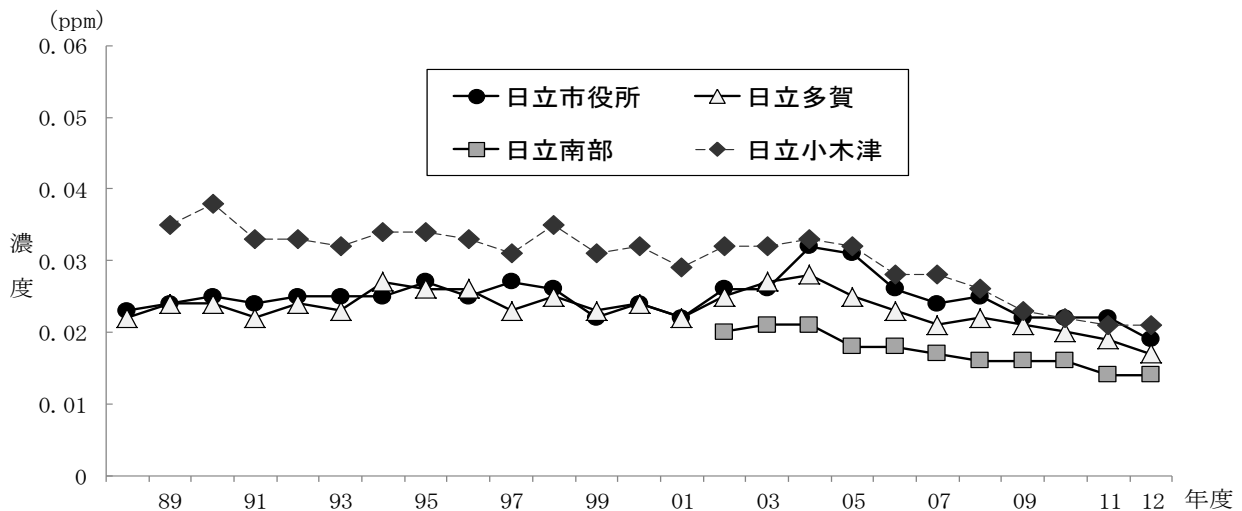
図1-4 二酸化窒素（日平均値の年間98%値）の経年変化
