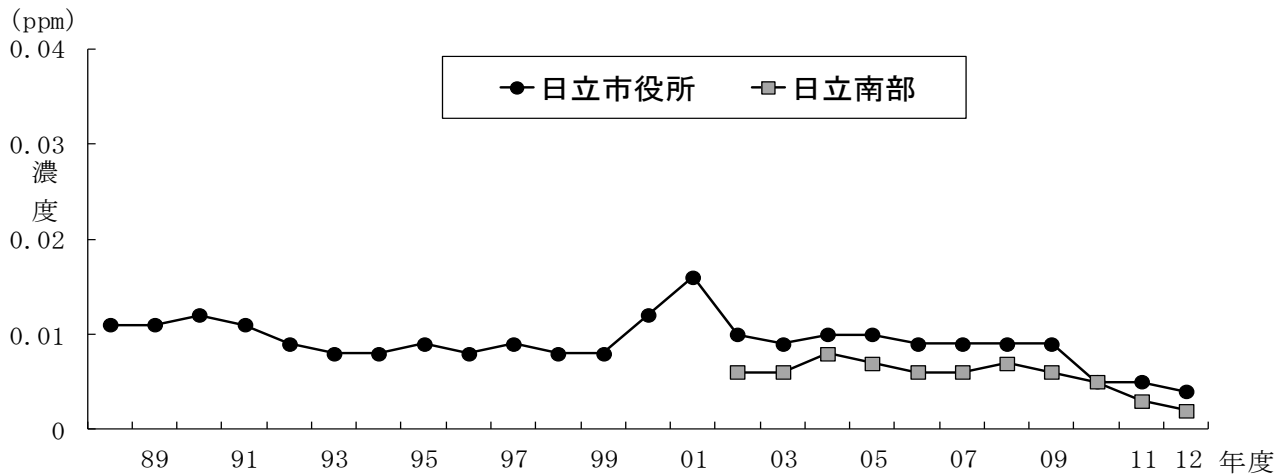
図1-2 二酸化硫黄（日平均値の年間2%除外値）の経年変化
