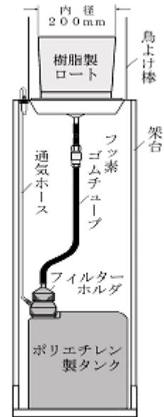
酸性雨ろ過式採取装置
