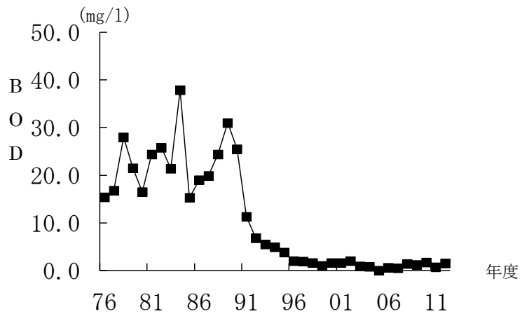
図1-9 BODの経年変化(金沢川)
