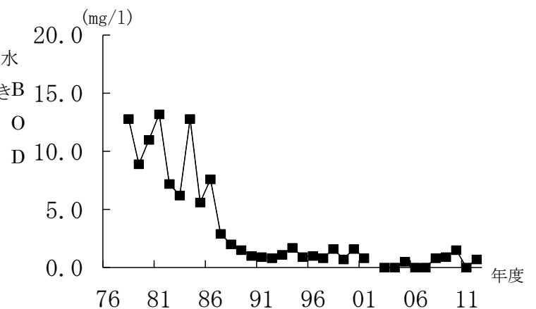
図1-4 BODの経年変化（北川）
