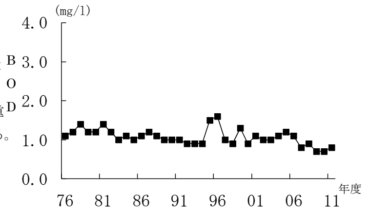
図1-2 BODの経年変化（久慈川）
