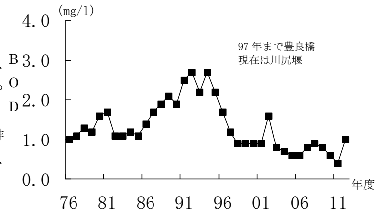
図1-3 BODの経年変化（十王川）
