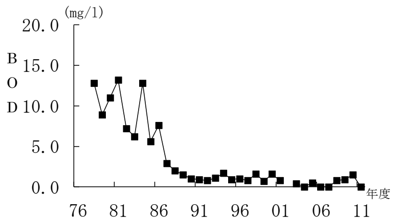
図1-4 BODの経年変化（北川）
