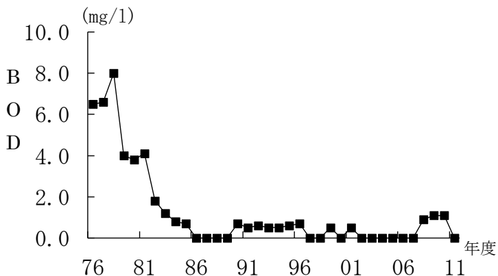
図1-7 BODの経年変化(鮎川)
