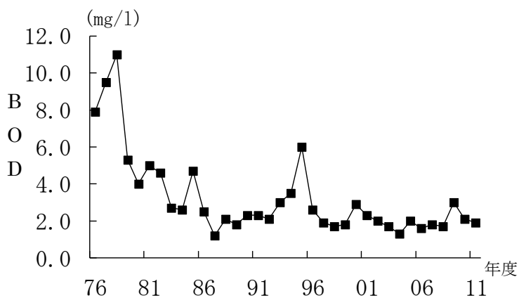
図1-5 BODの経年変化(宮田川)
