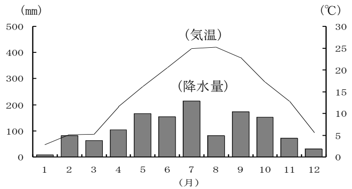
図1-2 気温と降水量の月変化 (2011年日立市役所観測所)
