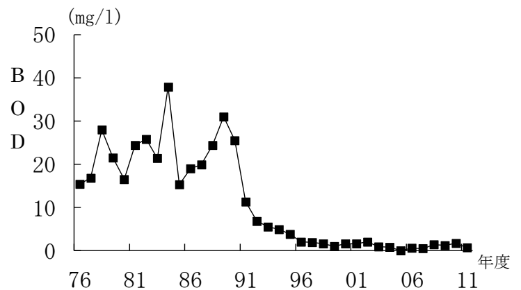
図1-9 BODの経年変化(金沢川)
