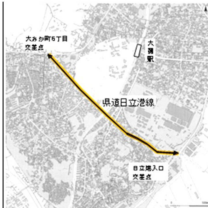
图 1-4 面的評価区間 (②県道日立港線)
