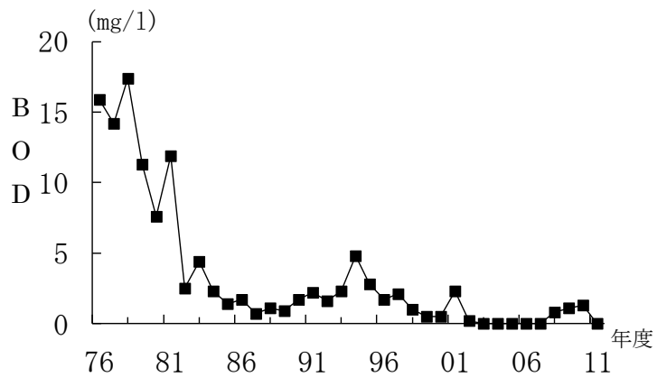
図1-8 BODの経年変化(桜川)
