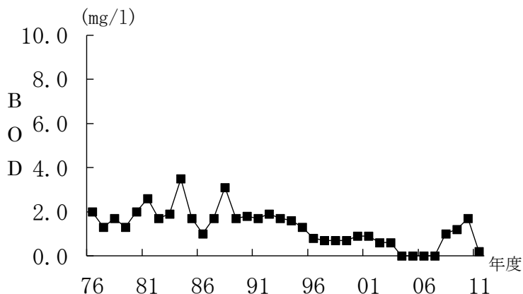
図1-6 BODの経年変化(東連津川)
