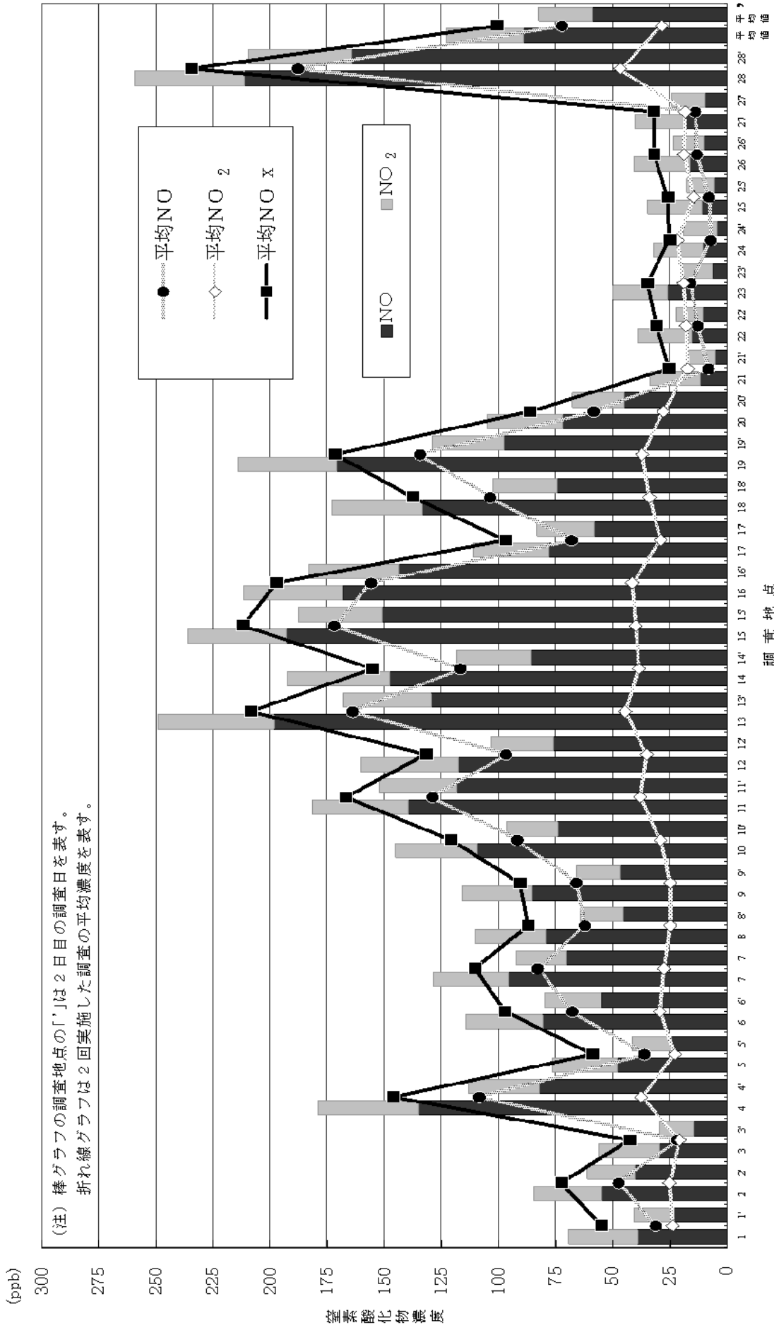
図1-4 窒素酸化物の濃度分布
