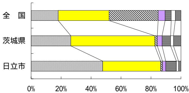
図2-1 騒音規制法に基づく特定施設数割合
