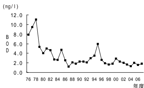
図1 - 5 BODの経年変化(宮田川)
