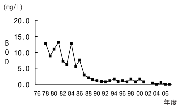
図1 - 4 BODの経年変化(北川)
