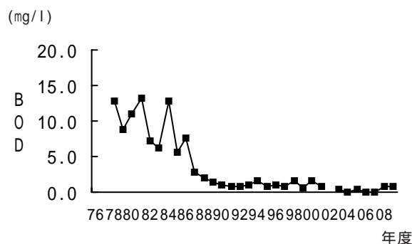
図1 - 4 BODの経年変化(北川)
