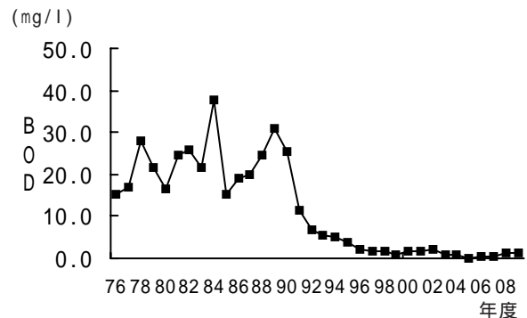
図1-9 BODの経年変化(金沢川)
