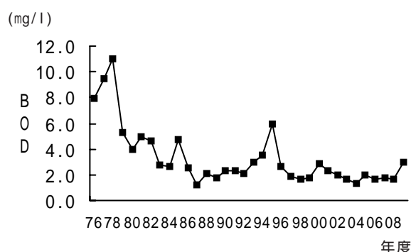
図1 - 5 BODの経年変化(宮田川)
