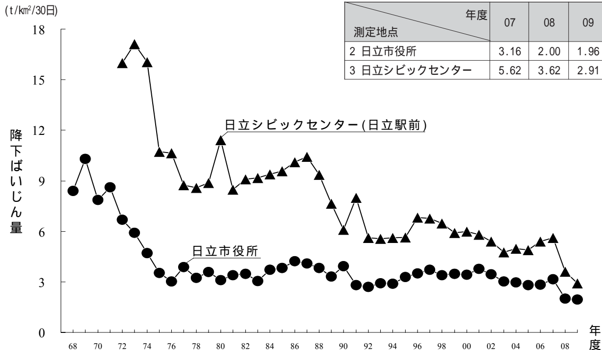
図1-6 降下ばいじん経年変化
