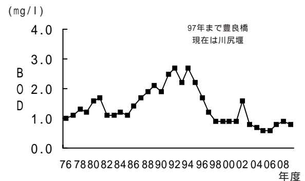
図1-3 BODの経年変化（十王川）
