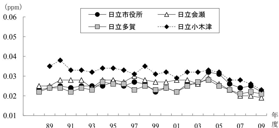
図1-4 二酸化窒素(日平均値の年間98%値)の経年変化
