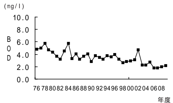
図1-10 BODの経年変化(茂宮川)
