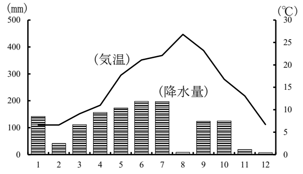
図1-2 気温と降水量の月変化 (2020年日立市役所観測所)
