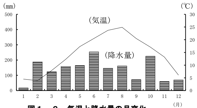
図1-2 気温と降水量の月変化 (2014年日立市役所観測所)
