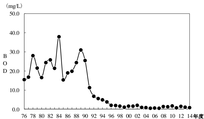
図 1-9 BODの経年変化(金沢川)
