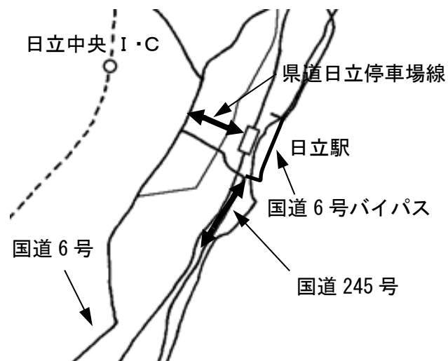
图 1-4 面的評価区間 (②国道 245 号、③県道日立停車場線)
