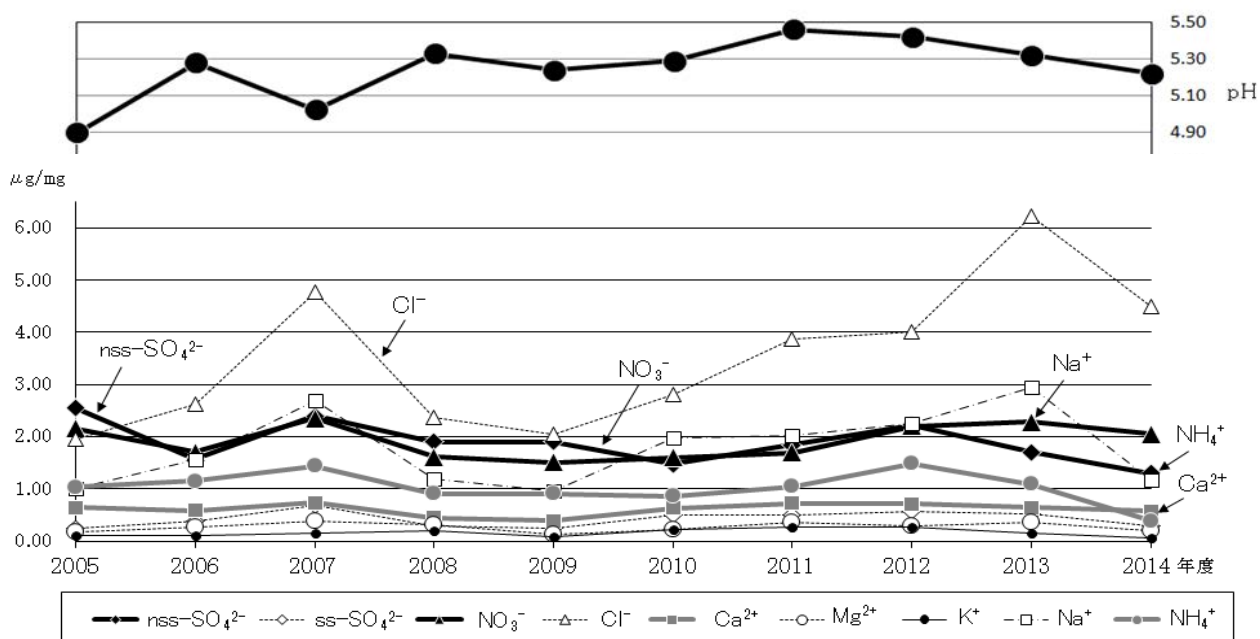
図1-1 pH・イオン成分の年間平均値の経年変化（日立市役所）
