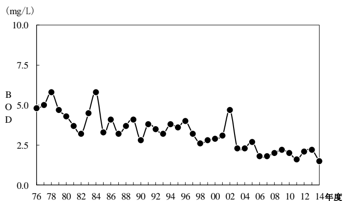
図 1-10 BODの経年変化(茂宮川)
